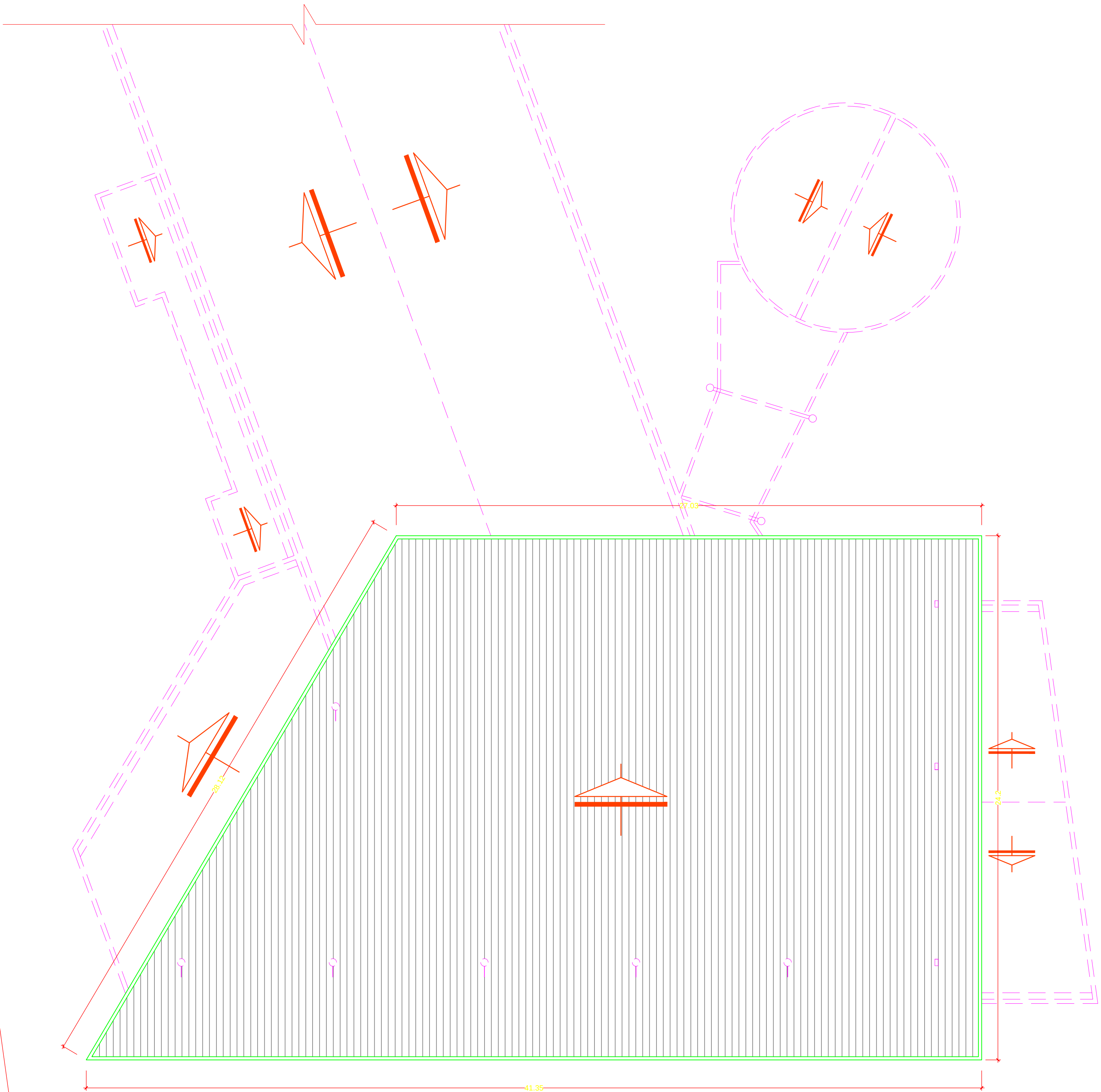
COBERTURA (ÁTRIO) ESC. 1:125
