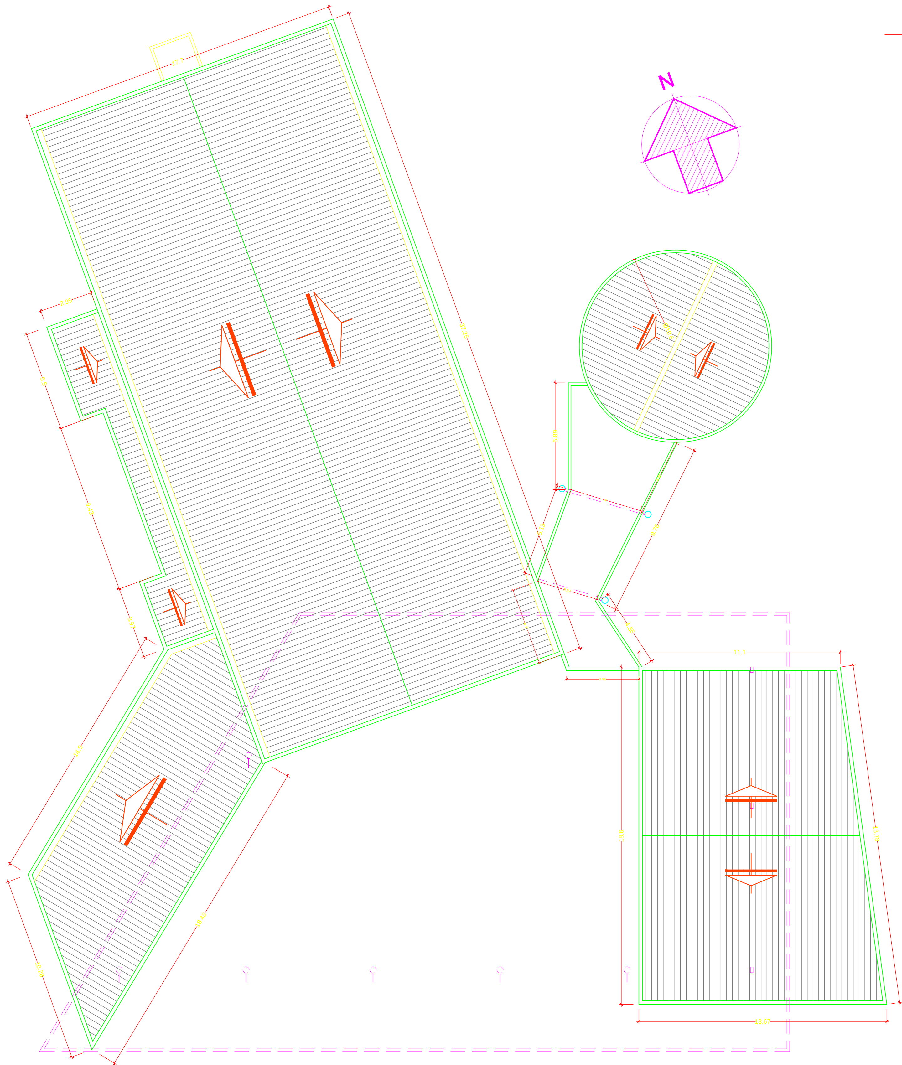
COBERTURA (PROJEÇÃO ABAIXO DO ÁTRIO) ESC. 1:125
