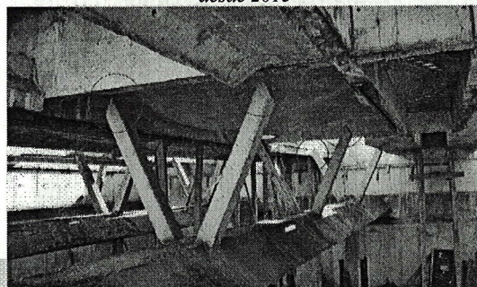
Figura 18 - Detalhe da obra do Reator UASB
