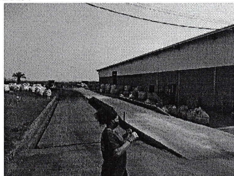
Figura 12: Área de operação da COOPERTAN, na imagem está demonstrada a balança rodoviária para pesagem dos caminhões.
