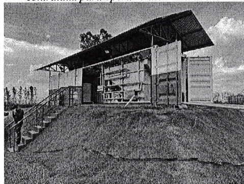
Figura 6: Estação de tratamento de chorume por flotor de ar dissolvido.
