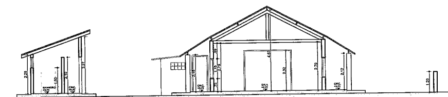
03 CORTE AA ESCALA 1/75
