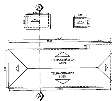
02 COBERTURA ESCALA 1/75
