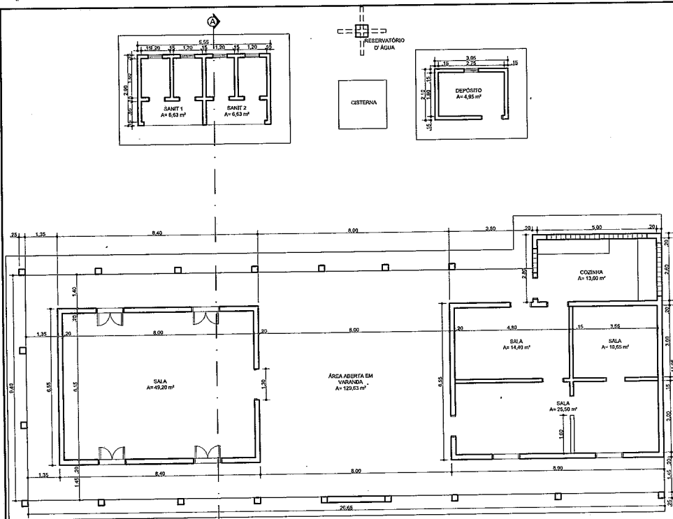
01 PLANTA BAIXA ESCALA 1/75
